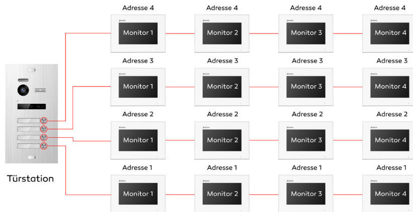
Adressen-Diagramm
