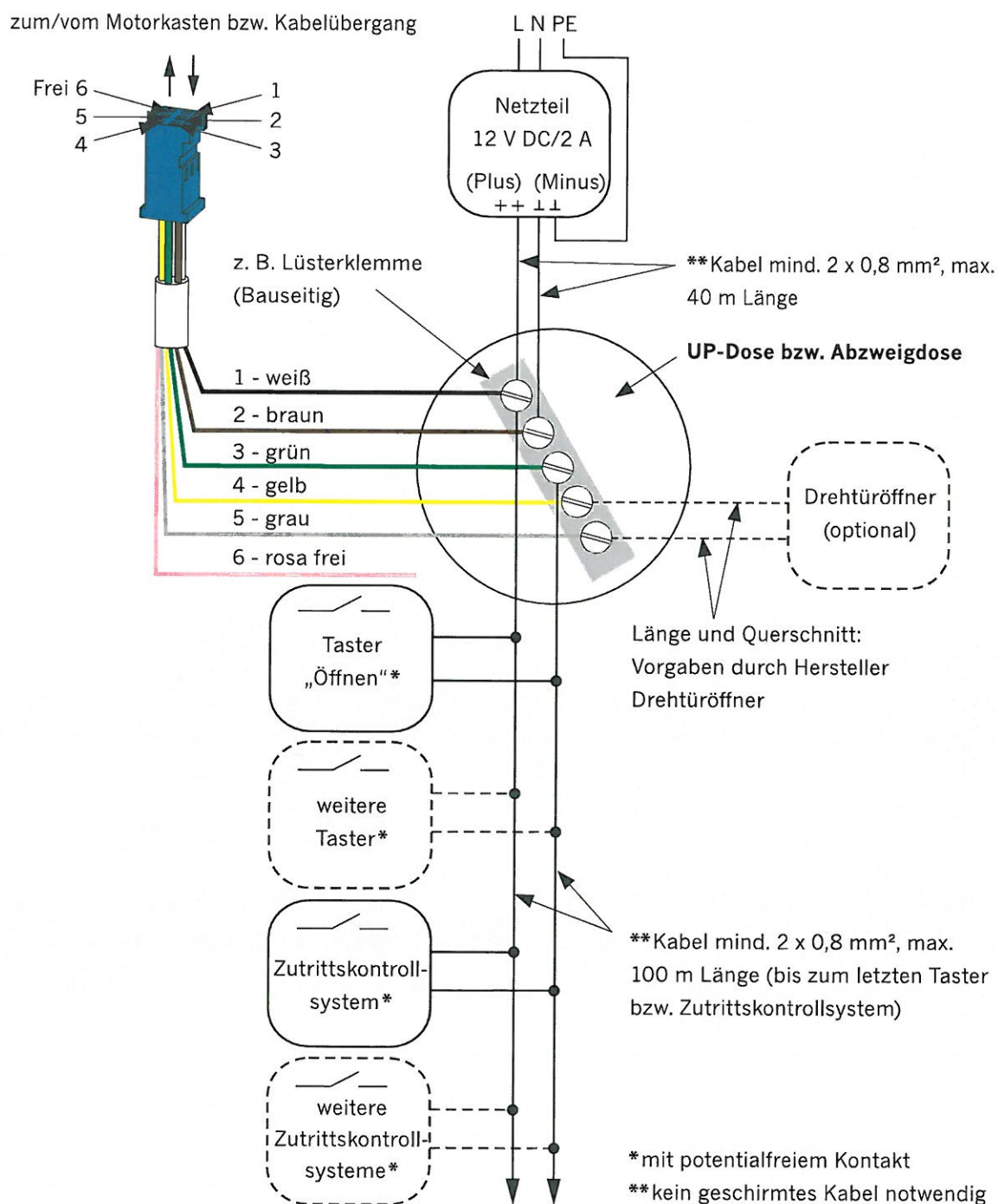
Abbildung 3.3.1-1: Allgemeiner Anschlussplan
